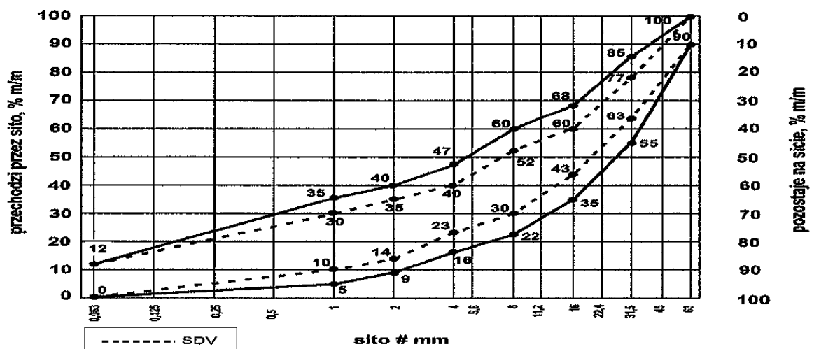
Rys. 3. Krzywe graniczne uziarnienia mieszanki kruszywa niezwiązanego 0/63 mm do warstw odcinającej
