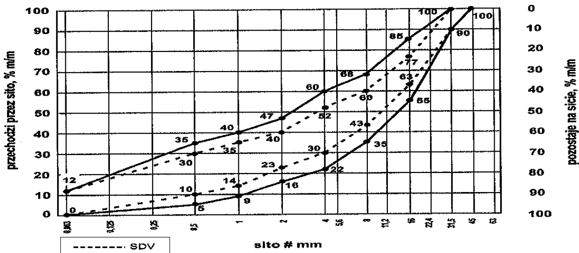
Rys. 1. Krzywe graniczne uziarnienia mieszanki kruszywa niezwiązanego 0/31,5 mm do warstw odcinającej
