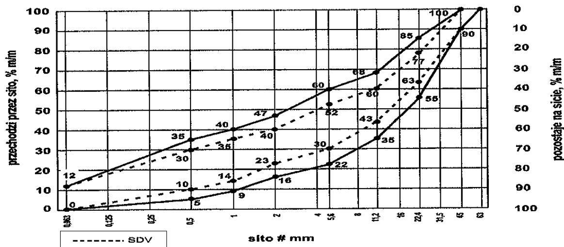
Rys. 2. Krzywe graniczne uziarnienia mieszanki kruszywa niezwiązanego 0/45 mm do warstw odcinającej
