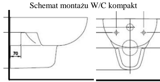
Miska ustępowa dla dzieci 6 letnich h= 300 mm
