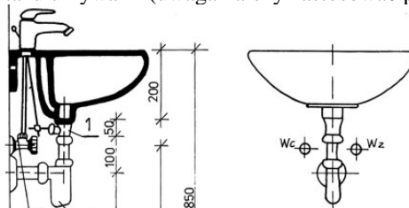
Schemat montażu umywalki
