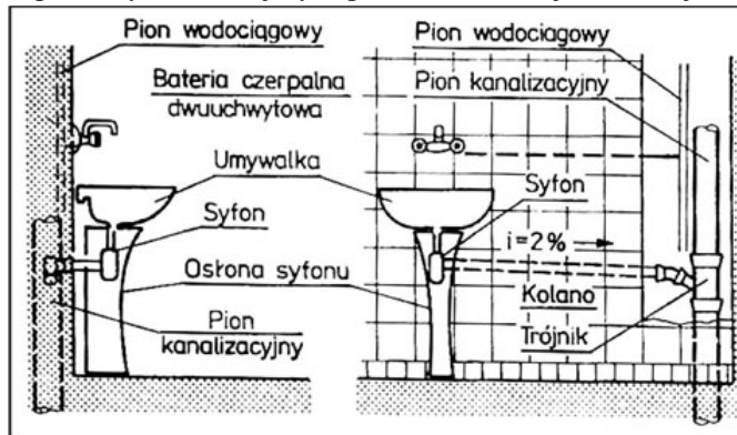
Schemat montażu umywalki (uwaga należy zastosować półpostument)
