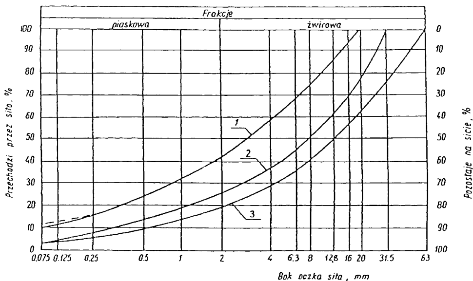
Rysunek 1. Pole dobrego uziarnienia
