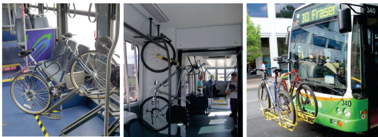
Rysunek 7a-7 Różne sposoby przewożenia rowerów środkami transportu zbiorowego: wewnątrz autobusu w uchwycie rowerowym, na wieszaku rowerowym, na bagażnikach rowerowych montowanych na autobusach
