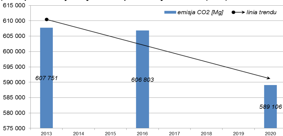
Wykres 14.1. Poziomy emisji CO 2 – w roku bazowym (2013), po uwzględnieniu już zrealizowanych działań (2016) oraz po realizacji wszystkich zaplanowanych działań (2020)
