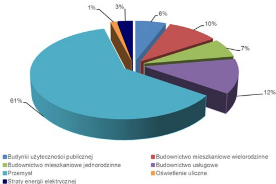
Wykres 6.21 Struktura zużycia energii elektrycznej w podsektorach sektora Budynki, obiekty i przemysł
