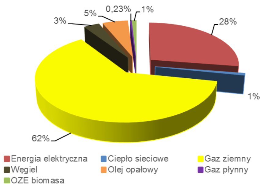
Wykres 5.11 Struktura zużycia energii w budynkach i obiektach przemysłowych
