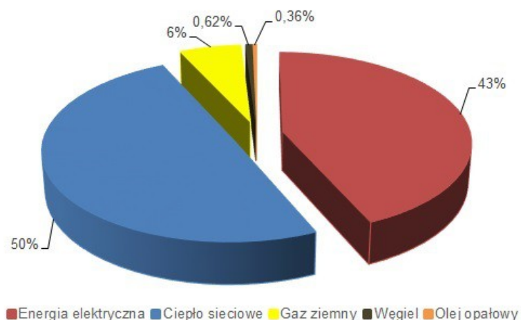
Wykres 6.24 Struktura emisji CO 2 w podsektorze obiektów użyteczności publicznej
