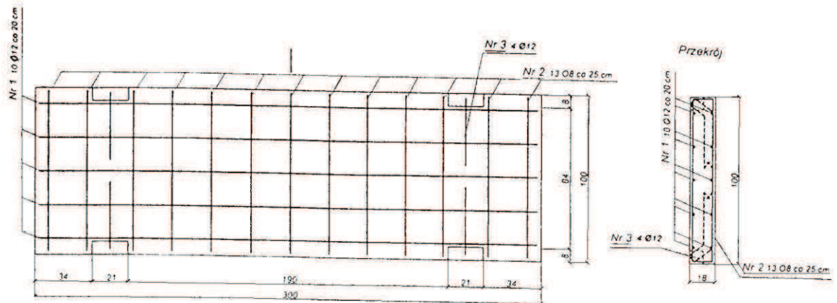
d) Płyta 3,0 \times 1,0 \times 0,18 m
