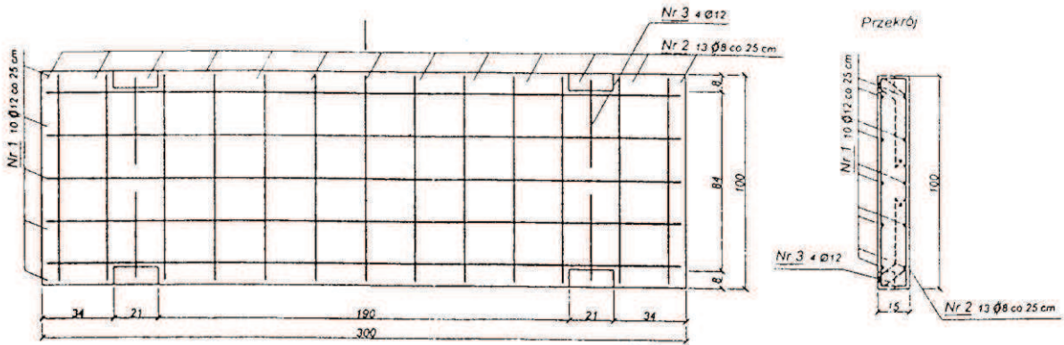
d) Płyta 3,0 \times 1,0 \times 0,18 m
