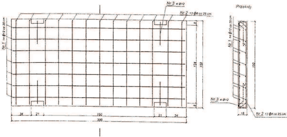
b) Płyta 3,0 \times 1,5 \times 0,15 m
