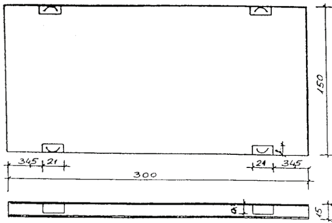
c) Płyta 3,0 \times 1,5 \times 0,18 m
