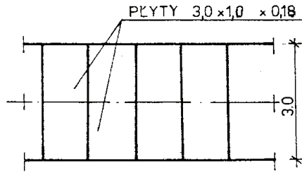
b) Płyty układane systemem płatowym
