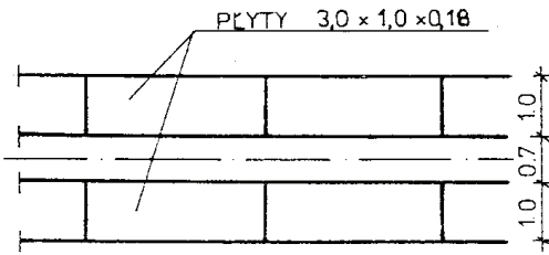
Rys. 2. Przykłady ułożenia płyt 3,0 \times 1,0 \times 0,18 m na jezdni jednopasowej a) Płyty układane systemem pasowym
